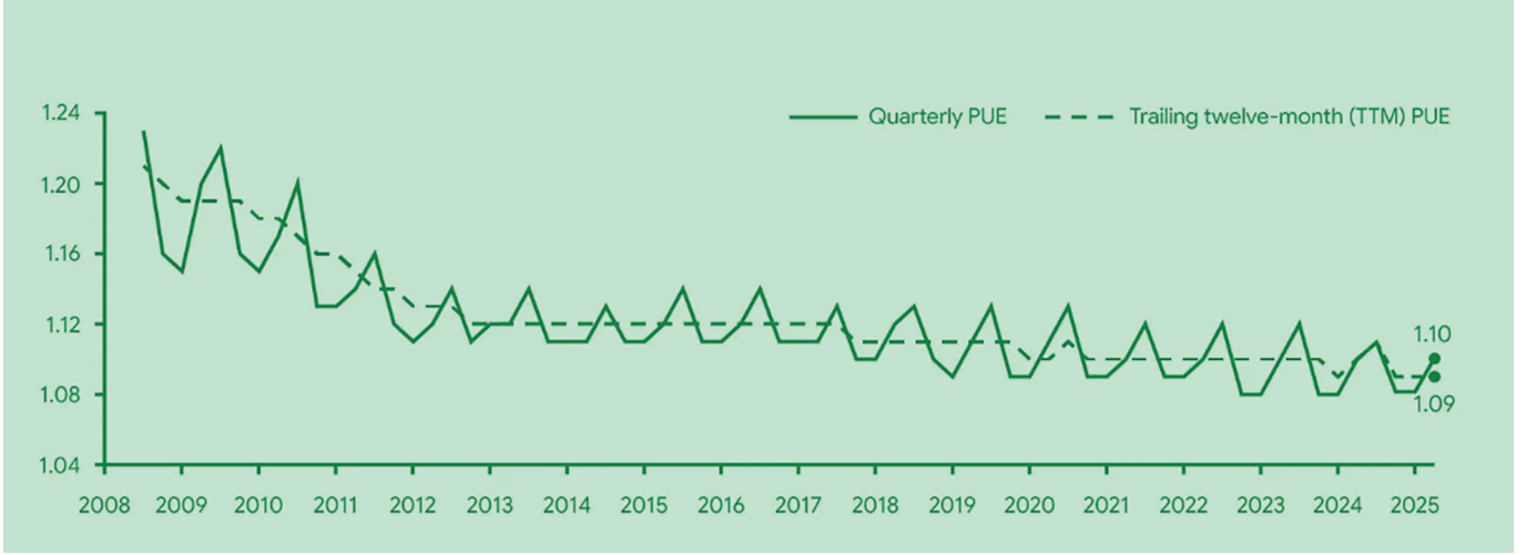
Grafik-8: Google veri merkezi PUE değerlerinin yıllar içindeki değişimi (Kaynak: Google Data Center PUE )
