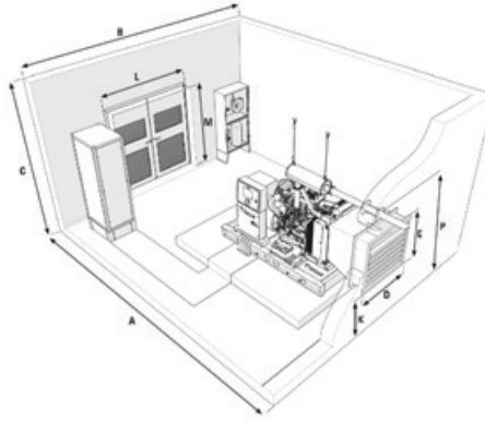
Örnek oda yerleşimi
