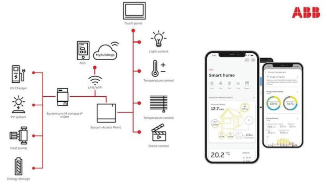
Şekil-3: Örnek bir akıllı ev projesinde entegre edilebilecek sistemlere ait örnek şema
